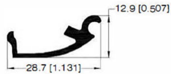
CANDADO BASICO 31611
