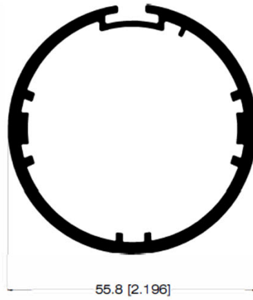
TUBO PARA CORTINA 32624
