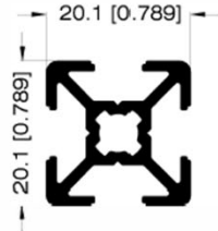
PERFIL 20mm X 20mm 32408
