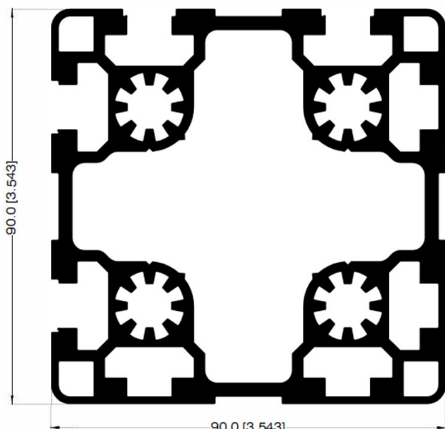
PERFIL 90mm X 90mm 32225
