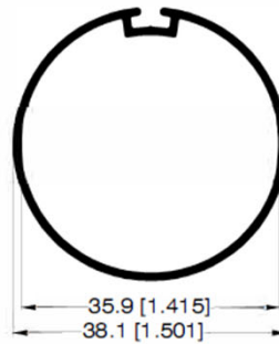
TUBO 32568
