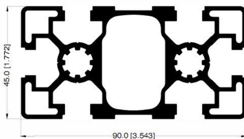
PERFIL 90mm X 45mm 32224
