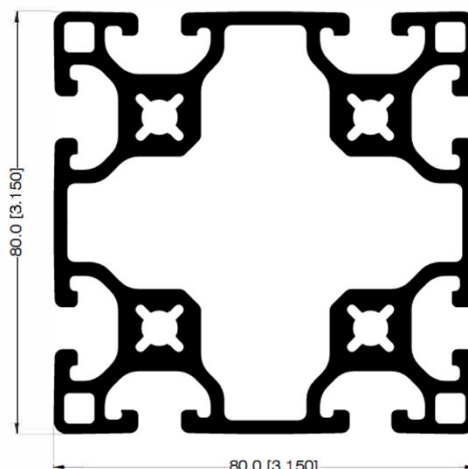
PERFIL 80mm X 80mm 32042
