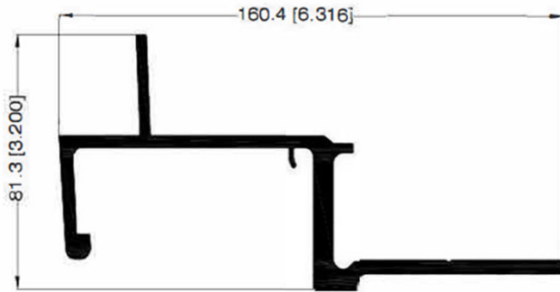
BORDA 32743
