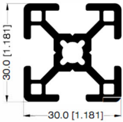
PERFIL 30mm X 30 mm 31696
