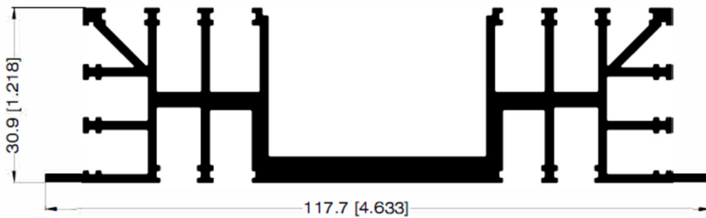
DISIPADOR 31816
