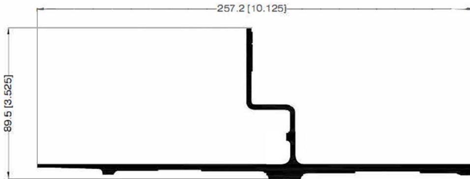
BORDA 32777
