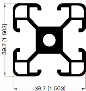
PERFIL 40mm X 40mm 32195
