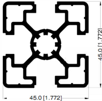
PERFIL 45mm X 45mm 32192
