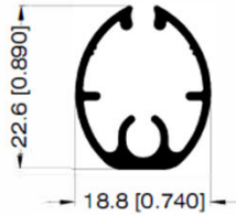
PERFIL CONTRAPESO 32052
