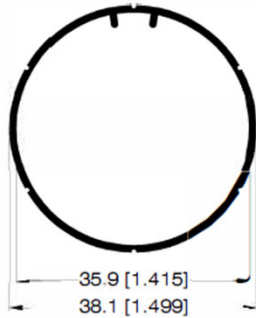
PERFIL CORTINERO 32442
