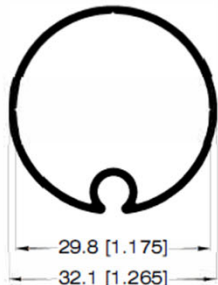
ROLUX CHICO 31083
