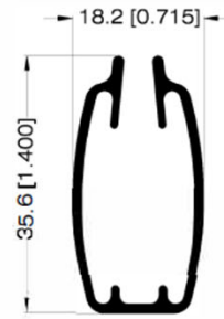
PERFIL CONTRAPESO 32196
