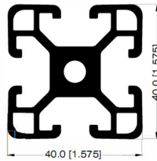
PERFIL 40mm X 40mm. 30460
