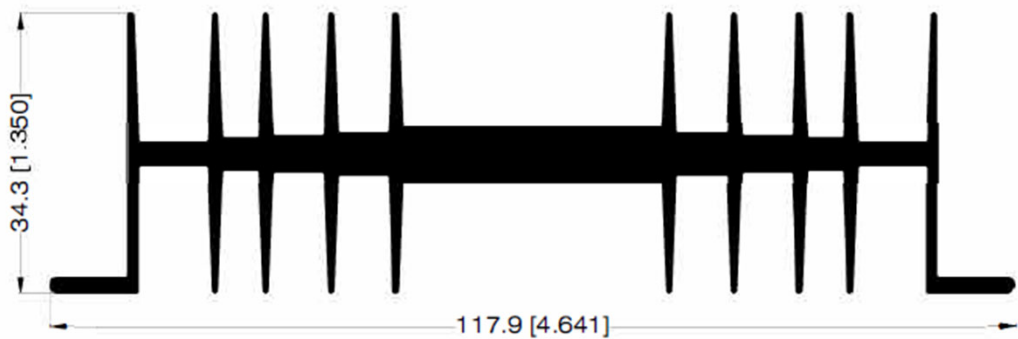
DISIPADOR 31928
