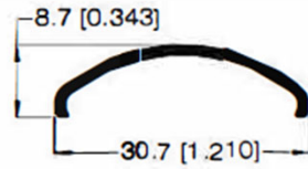
MOLDURA ACOPLABLE 30249
