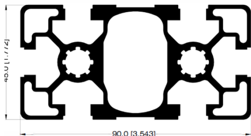
PERFIL 45mm X 90mm 32841
