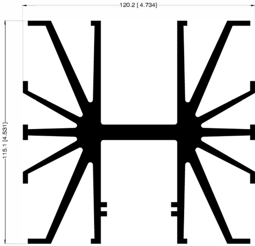
DISIPADOR 31927
