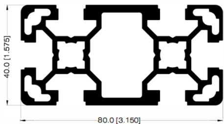
PERFIL 40mm X 80mm 32843
