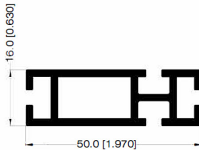
LARGUERO PARA MAMPARA 30247
