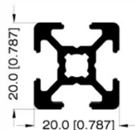
PERFIL 20mm X 20mm 32845
