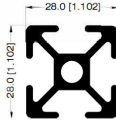
PERFIL 28mm X 28mm 30762
