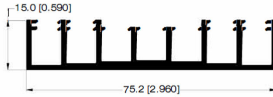
DISIPADOR 31750
