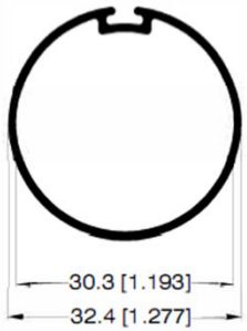
PERFIL CORTINERO 32443
