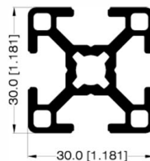
PERFIL 30mm X 30mm 32842
