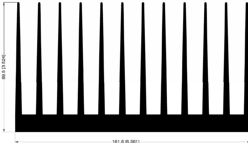
DISIPADOR 32021
