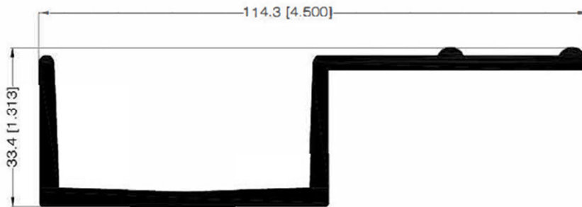
PERFIL BORDA DE 4.500" X 1.313" 30169
