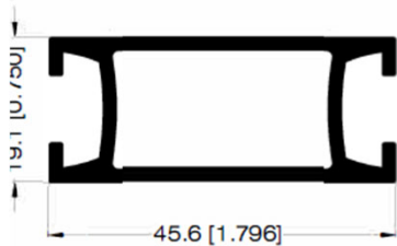
LARGUERO PARA MAMPARA 30263
