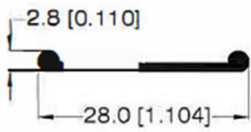
MOLDURA ACOPLABLE 30248
