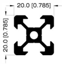
PERFIL 20mm X 20mm 32447
