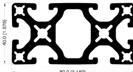
PERFIL 80mm X 40mm 31460
