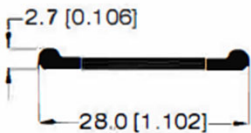
MOLDURA ACOPLABLE 30996
