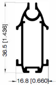
PERFIL RULOX 32005
