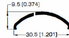
MOLDURA ACOPLABLE 30995
