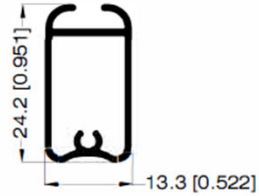
C. NEOLUX II 32267
