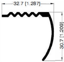
PERFIL PARA ESTRIBO 31054
