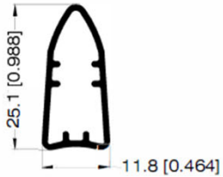
PERFIL PARA CORTINA 32266
