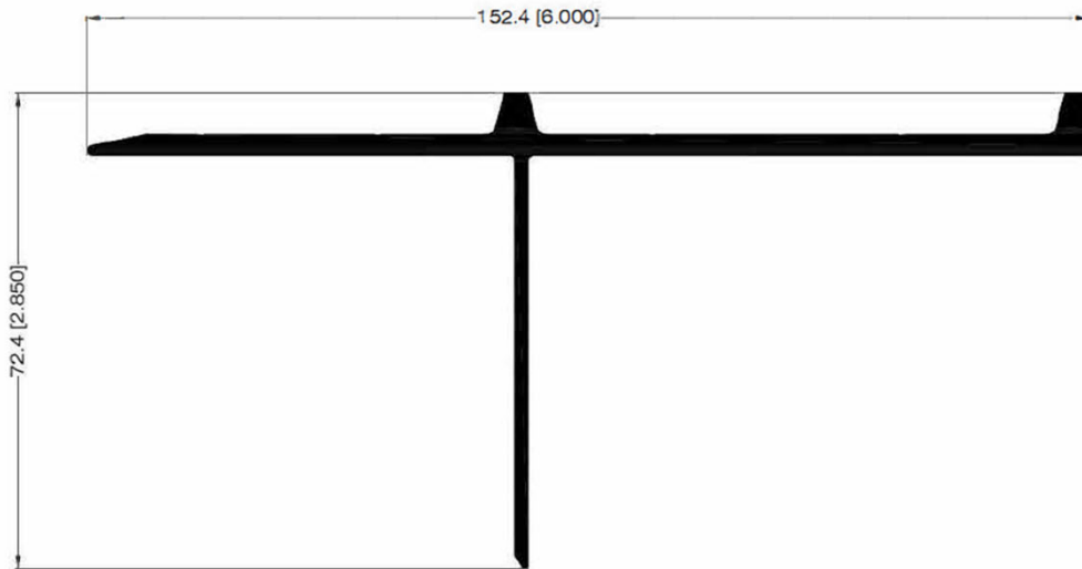
BORDA INFERIOR 30706
