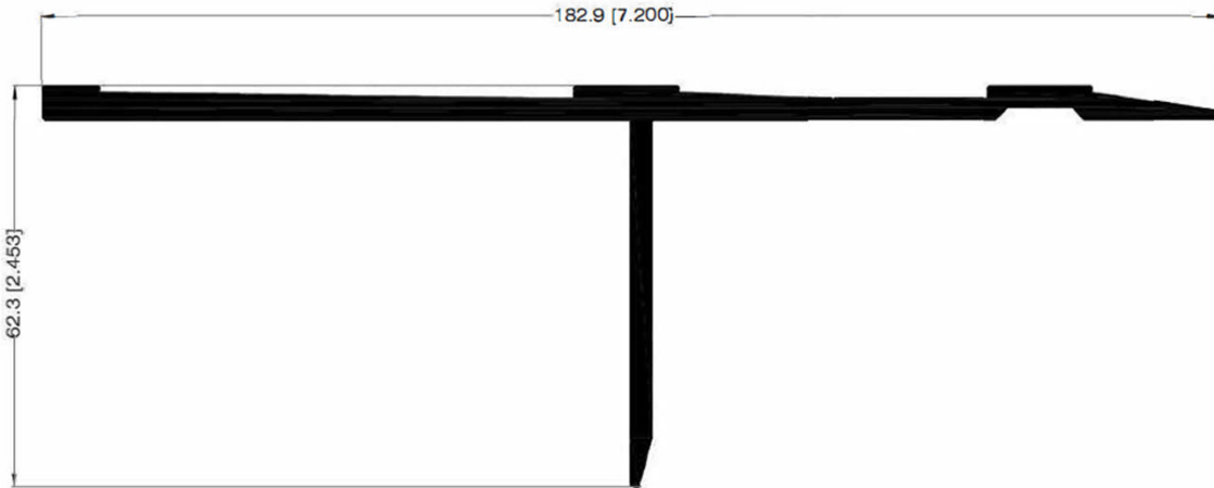
BORDA INFERIOR 31261
