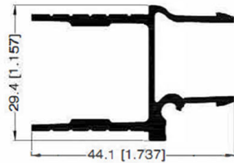
MACHO BASICO 31613
