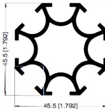
BARROTE PARA MAMPARA 30264
