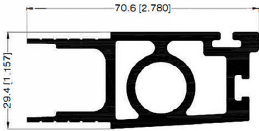
PORTACAÑUELA 31615
