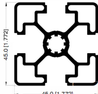
PERFIL 45mm X 45mm 32194
