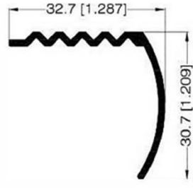
PERFIL PARA ESTRIBO 30997
