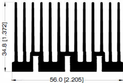
DISIPADOR 31821
