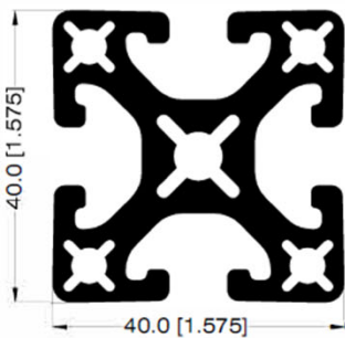
PERFIL 40 mm X 40mm 31458
