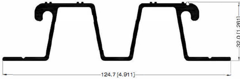
PERFIL PARA PISO 32774
