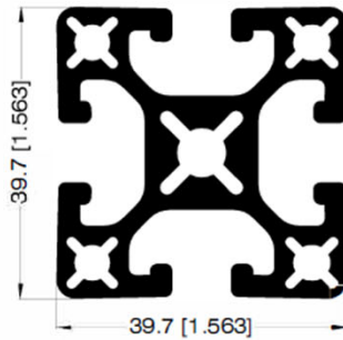
PERFIL 40mm X 40 mm 32529
