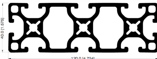
PERFIL 120mm X 40mm 32379
