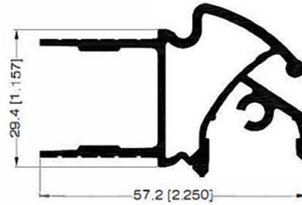
PERFIL HEMBRA BASICO 31612
