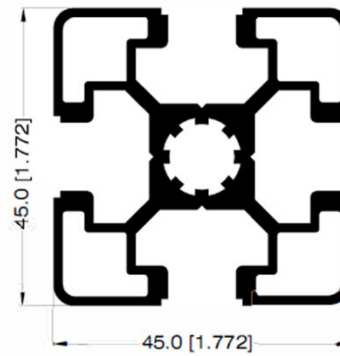
PERFIL 45 mm X 45mm 31673
