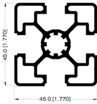
PERFIL 45 mm X 45mm 32422
