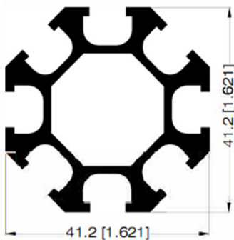
BARROTE PARA MAMPARA 30663
