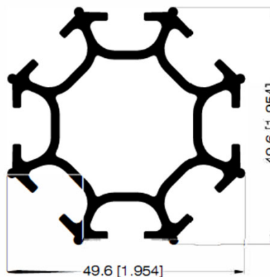
BARROTE PARA MAMPARA 30464
