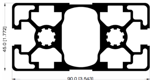
PERFIL 45mm X 90mm L 32850
