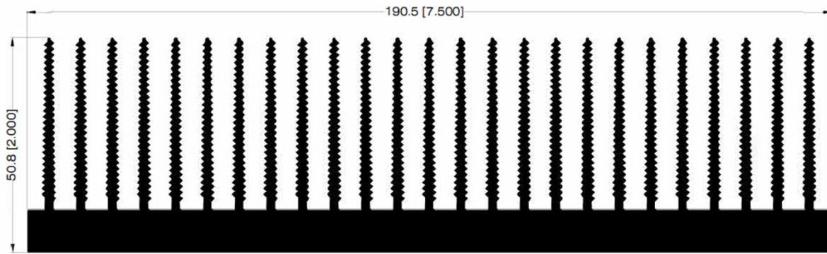
DISIPADOR 32261
