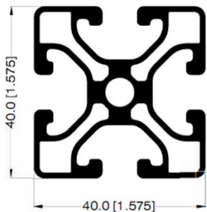
PERFIL 40mm X 40mm 32510
